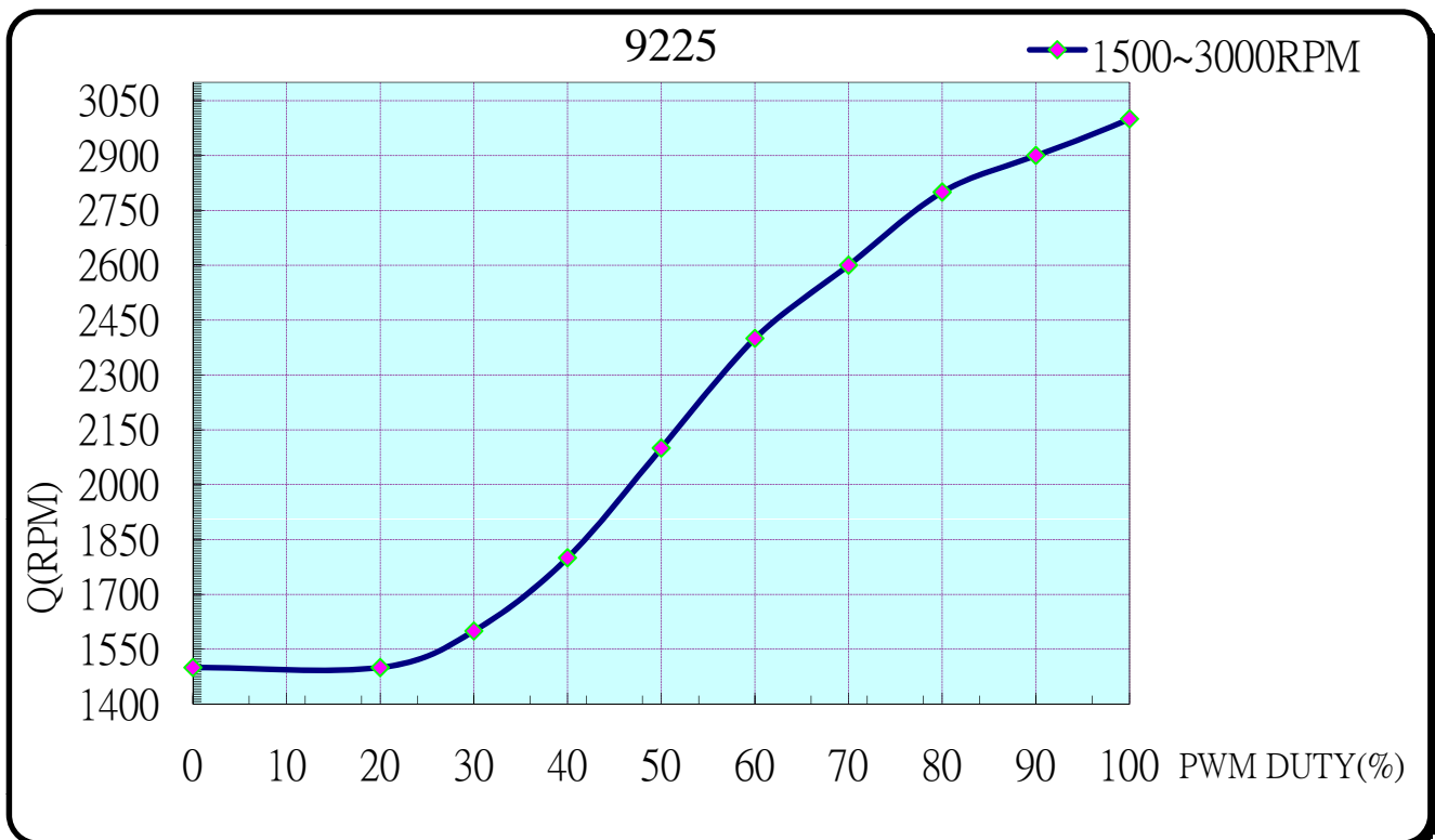
Fan PWM Curve
